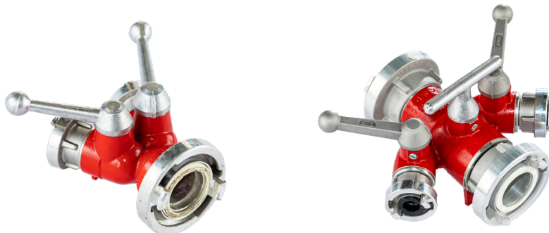
Abbildung 45: links C-DD-Verteiler, rechts C-DCD-Verteiler, beide mit Kugelhähnen
